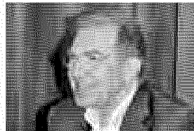
FRANCO ANTOCI
