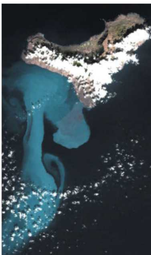
LA MANCHA VOLCÁNICA, MÁS GRANDE QUE EL HIERRO. Los restos de la erupción de El Hierro cubren ya una superficie del océano superior a la de la isla. Aunque afecta a la fauna, también creará un abono gigantesco, creen los expertos. / SATELITE DEMOS-1
